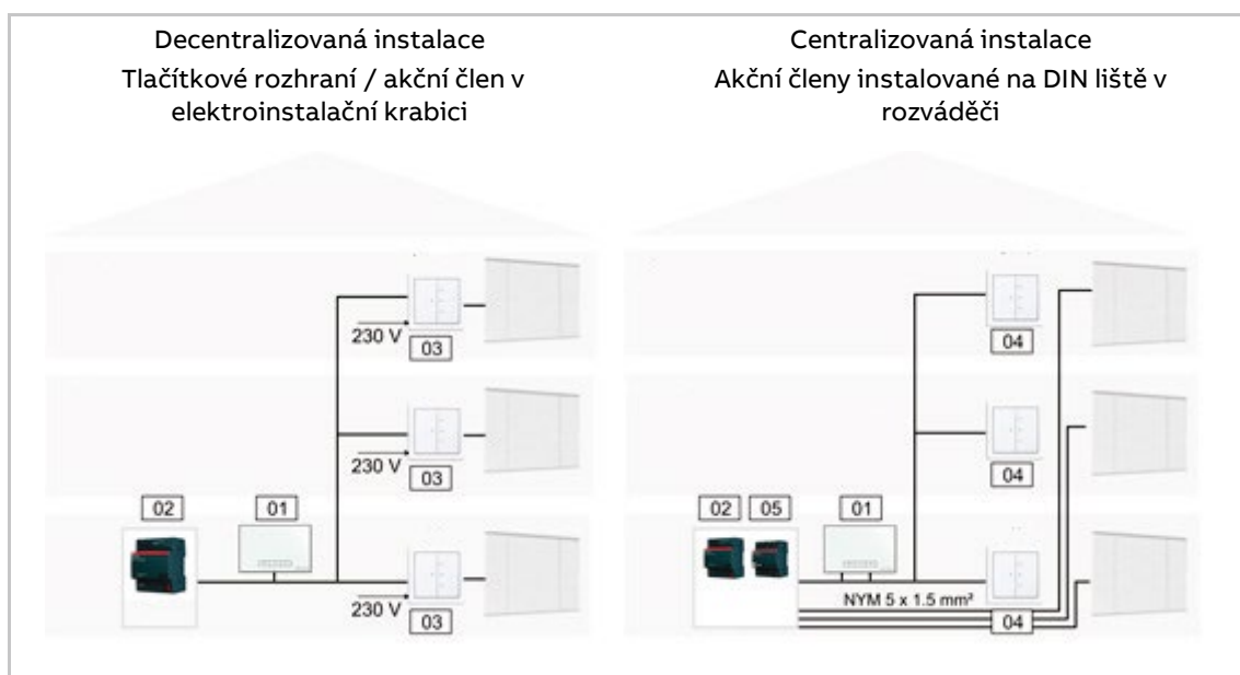
Obr. 2: Instalace se sběrniceovým kabelem
