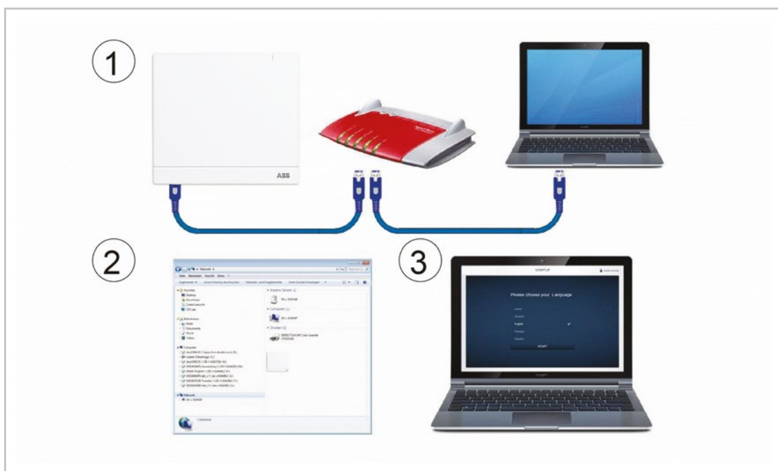
Obr. 20: Připojení PC pomocí datového kabelu a routeru
