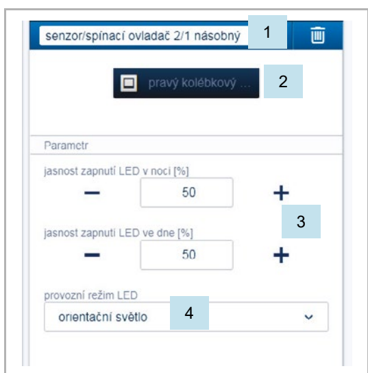
Obr. 47: Nastavení kolébky
