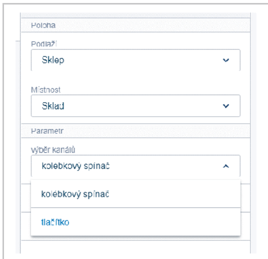
Obr. 42: Funkce „Tlačítko“
