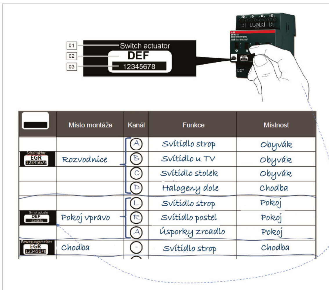
Obr. 16: Tabulka přístrojů
