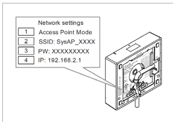
Obr. 17: Síťové informace na zadní části systémového modulu
