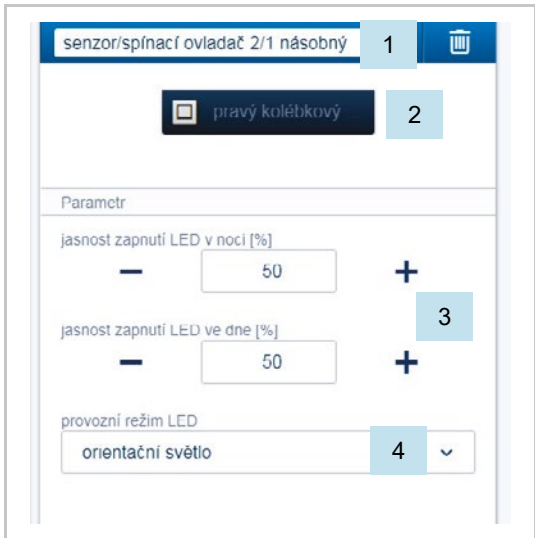
Obr. 58: Nastavení kolébky
