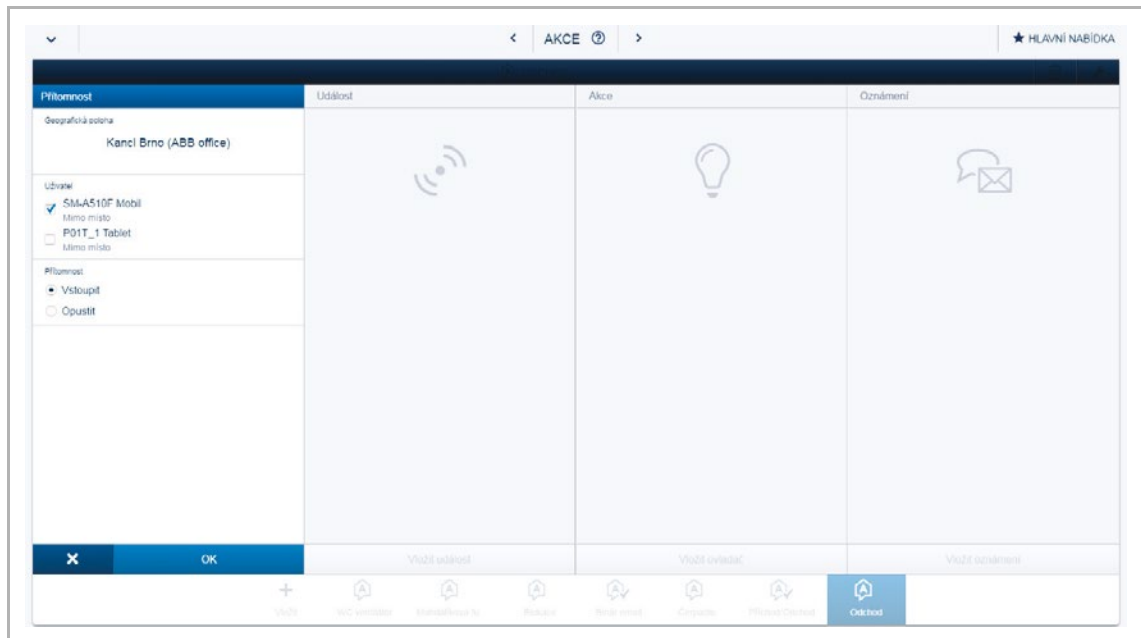
Obr. 82: Vytvoření akcí
